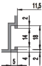
Frame groove 14/18
